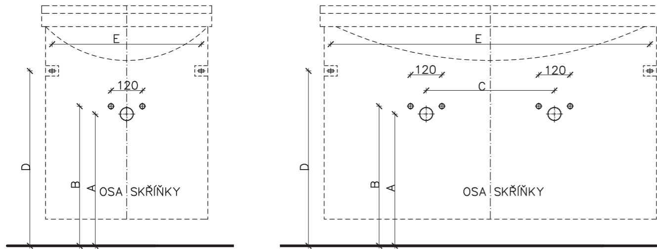
A – výška odpadu, B – výška vody, C – rozteč odpadů u dvojumyvadel, D – výška uchycení skříňky, E – rozteč uchycení skříňky = vnitřní šířka skř. – 50 mm, E – rozteč uchycení skříňky
